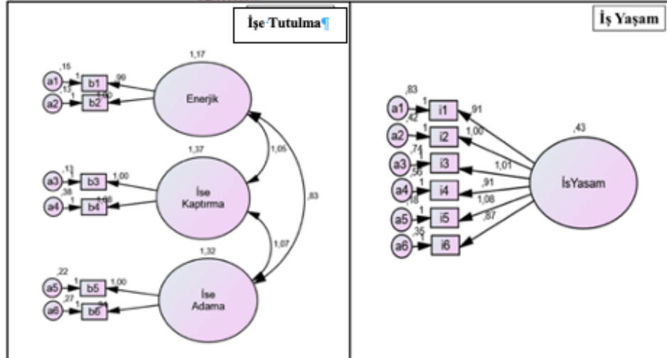
Şekil 2. DFA Faktör Yapıları
