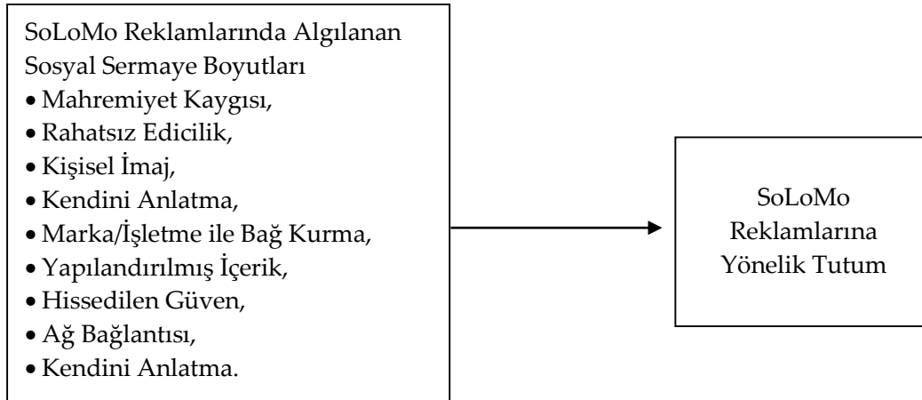
Şekil 1. Araştırma Modeli
