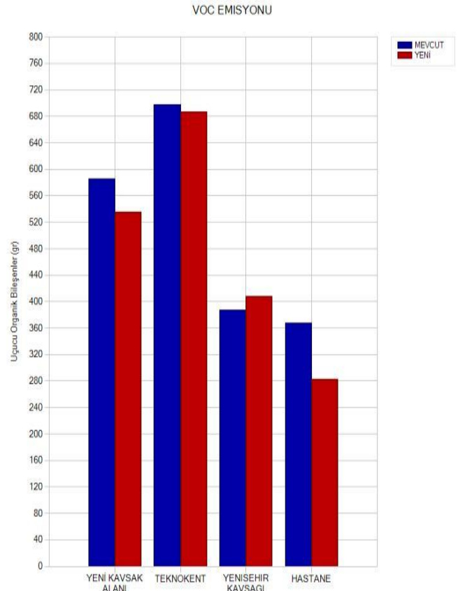
Şekil 13. VOC emisyonları
