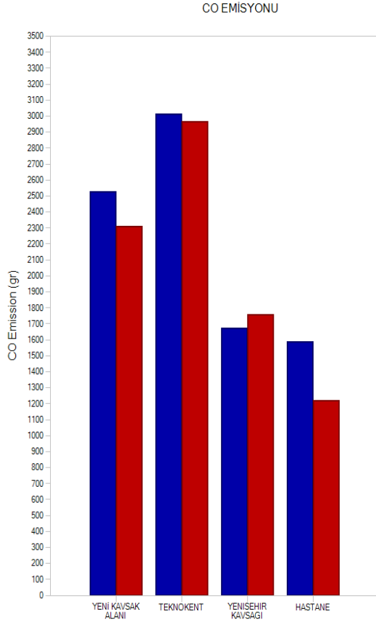
Şekil 11. CO emisyonları.
