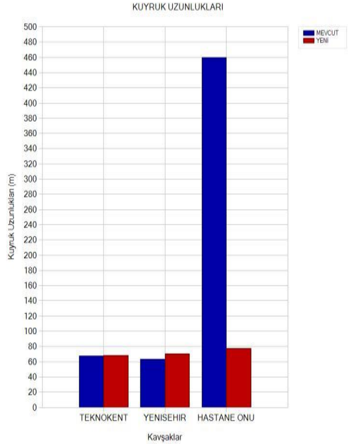
Şekil 10. Kuyruk uzunlukları.
