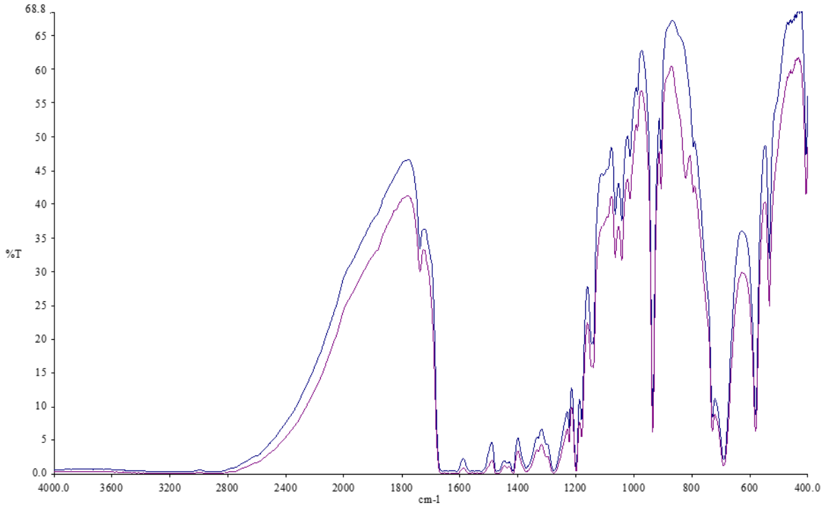
Şekil 5. BAA-Poliamit membranın (Kırmızı) ve Orijinal Poliamit destek tabakasının (Mavi) FTIR spektrumları
