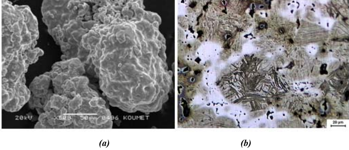
Şekil 7. (a) Sinter çeliklerin üretiminde kullanılan HP1 tozları; SEM görüntüsü. (b) Preslenmiş ve sonrasında sinterlenmiş çeliğe ait mikroyapı, Işık mikroskop görüntüsü.
