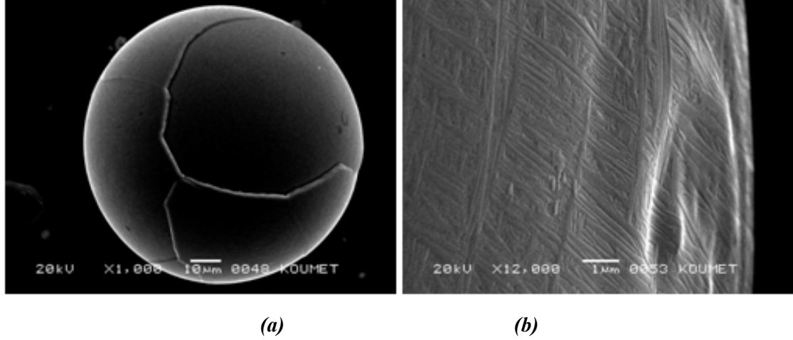
Şekil 6. Atomize tozlara ait tarama elektron mikroskop (SEM) görüntü örnekleri.
