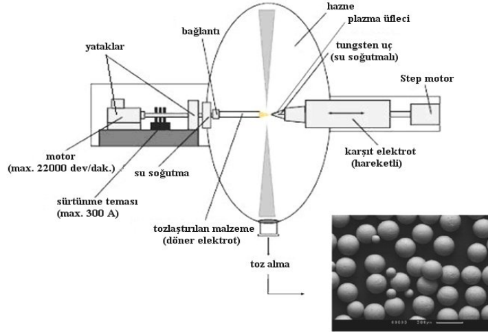
Şekil 3. Plazma destekli dönel elektrot sistemin şematik gösterimi.
