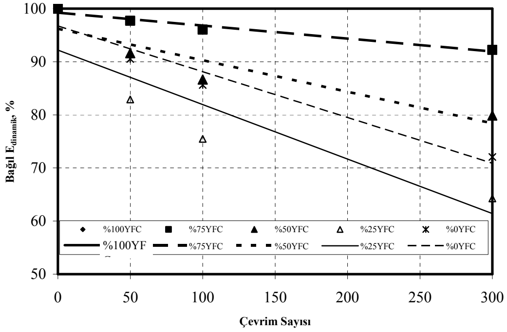
Şekil 9. \text{Na}_2\text{SiO}_3 (III) ile aktive edilen harçların dinamik elastisite modülleri
