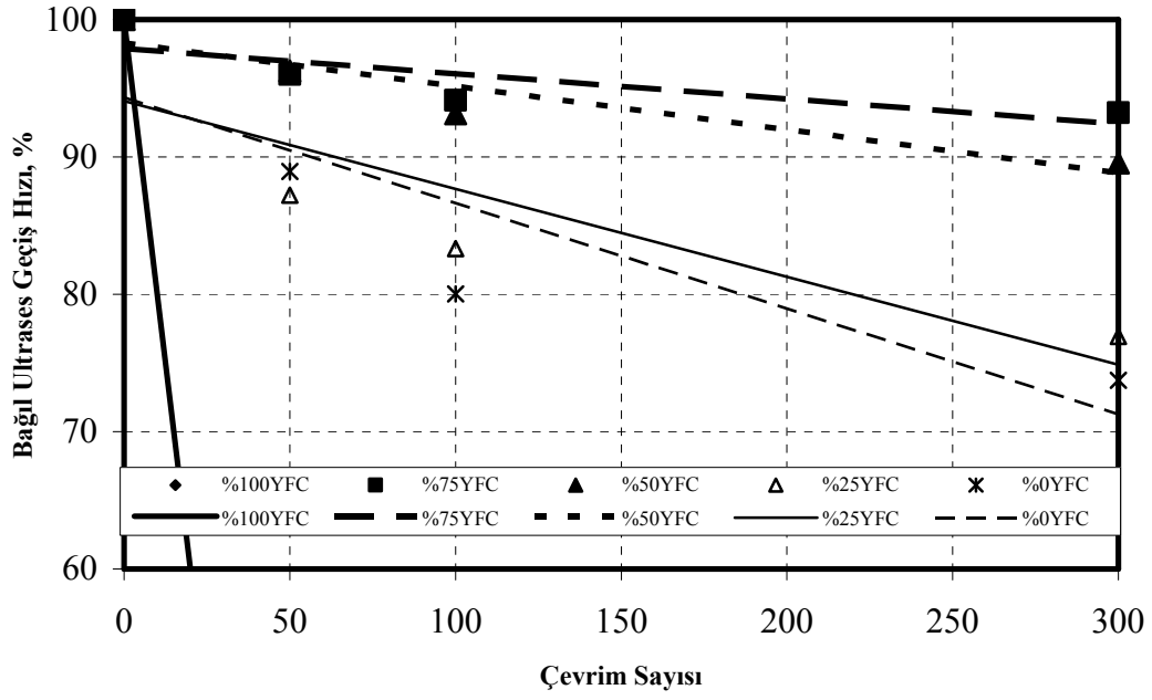
Şekil 6. \text{Na}_2\text{SiO}_3 (III) ile aktive edilen harçların ultrases geçiş hızı deney sonuçları
