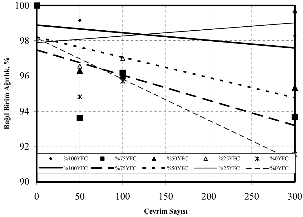
Şekil 2. \text{NaOH}+\text{Na}_2\text{SiO}_3 (II) ile aktive edilen harçların birim ağırlık deney sonuçları
