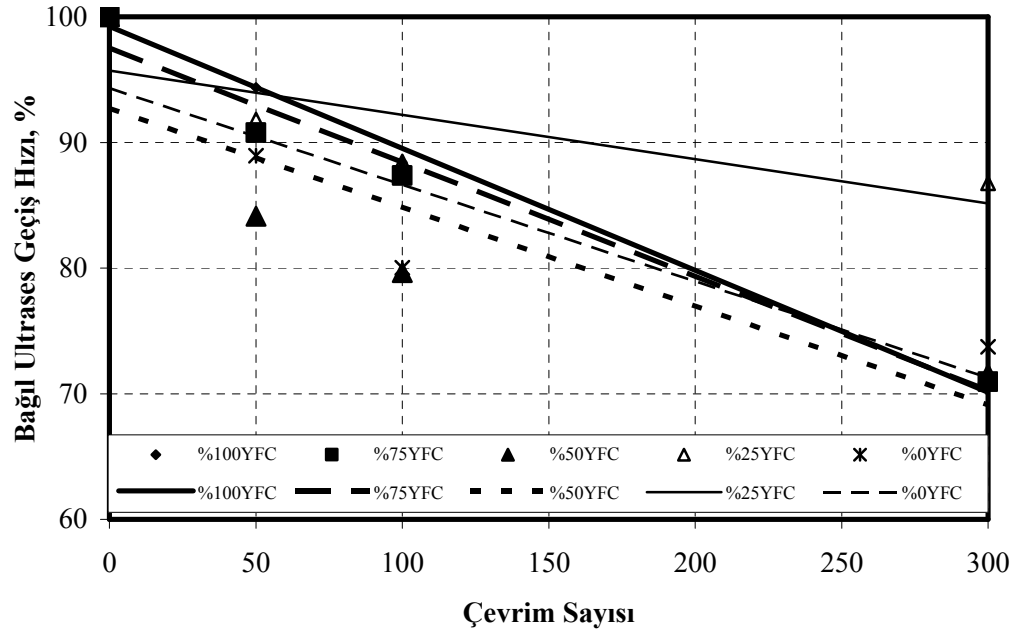
Şekil 4. \text{NaOH}+\text{Na}_2\text{CO}_3 (I) ile aktive edilen harçların ultrases deneyi sonuçları
