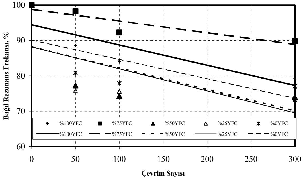
Şekil 11. \text{NaOH}+\text{Na}_2\text{SiO}_3 (II) ile aktive edilen harçların rezonans frekansı sonuçları
