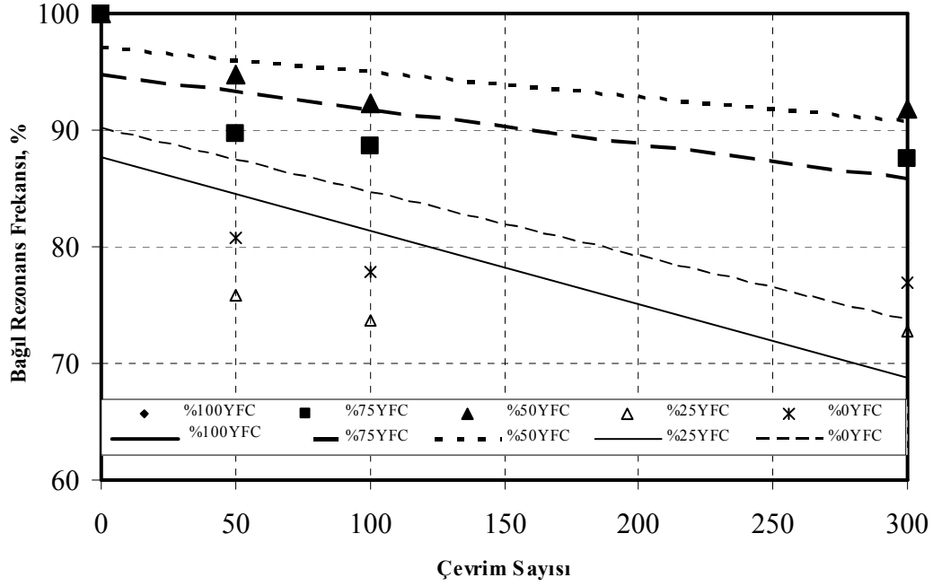
Şekil 12. \text{Na}_2\text{SiO}_3 (III) ile aktive edilen harçların rezonans frekansı deney sonuçları
