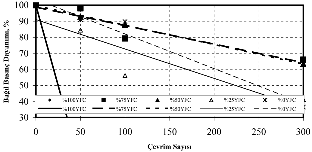
Şekil 15. \text{Na}_2\text{SiO}_3 (III) ile aktive edilen harçların basınç dayanımı deney sonuçları
