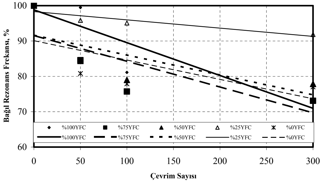
Şekil 10. \text{NaOH}+\text{Na}_2\text{CO}_3 (I) ile aktive edilen harçların rezonans frekansı sonuçları
