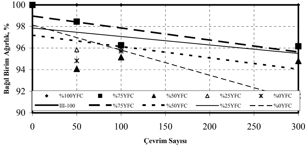
Şekil 3. \text{Na}_2\text{SiO}_3 (III) ile aktive edilen harçların birim ağırlık deney sonuçları
