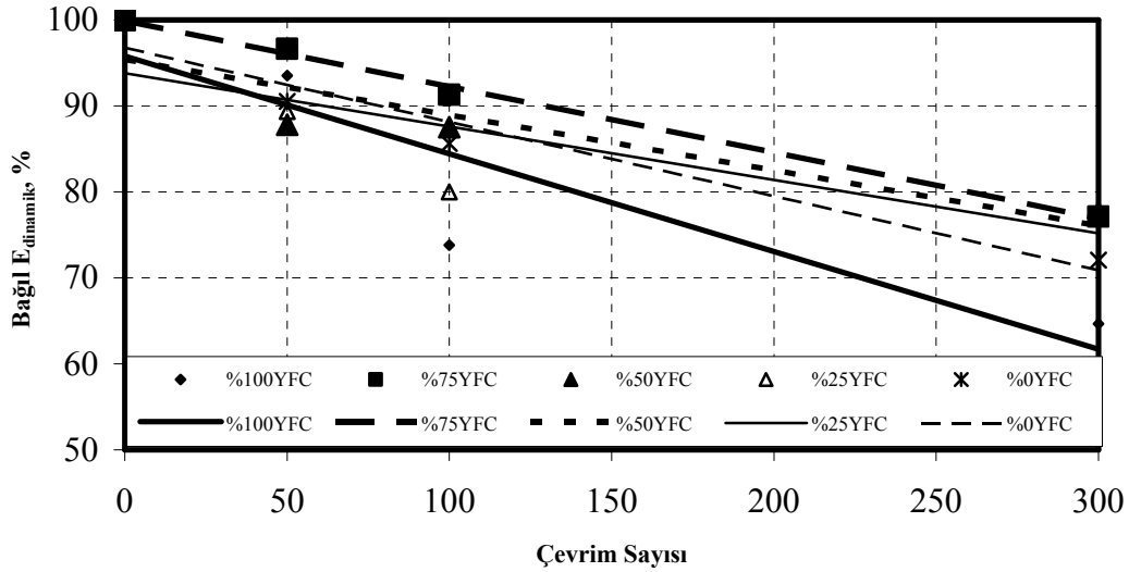
Şekil 8. \text{NaOH}+\text{Na}_2\text{SiO}_3 (II) ile aktive edilen harçların dinamik elastisite modülleri
