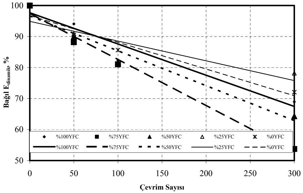
Şekil 7. \text{NaOH}+\text{Na}_2\text{CO}_3 (I) ile aktive edilen harçların dinamik elastisite modülleri
