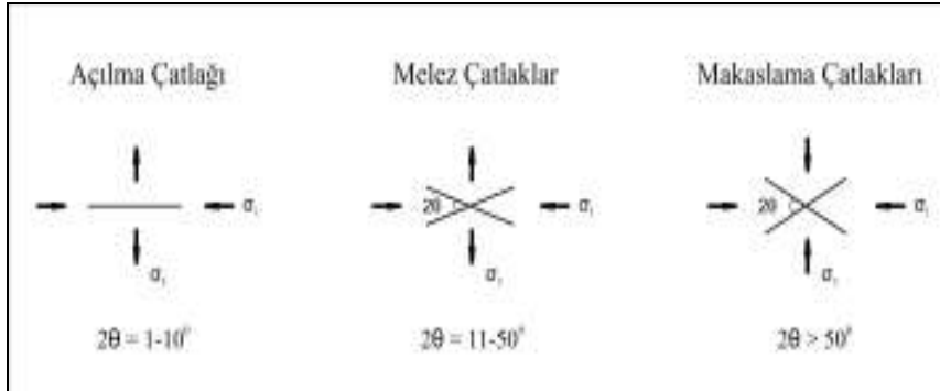
Şekil 5. Farklı gerilme koşullarında oluşan çatlak tipleri ( \sigma_1 en büyük ve \sigma_3 en küçük asal gerilme yönlerini göstermektedir) [41].
