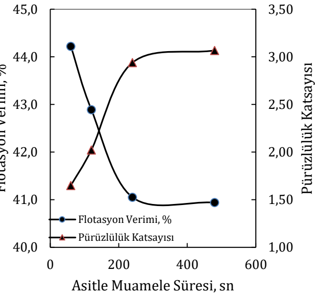
Şekil 9. Asitle Muamele Edildikten Sonra Öğütülen Cam Kürelerinin Flotasyonunda Pürüzlülük Katsayısının Etkisi ( 10^{-4} M kollektör konsantrasyonunda, pH: 7,1, 10 ppm MIBC eklentisi, Asitle Muamele Süreleri: 60, 120, 240, 480 sn)
