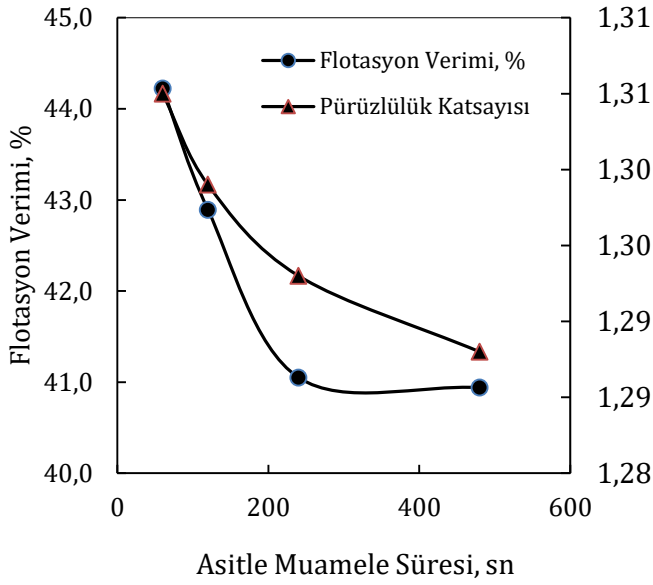
Şekil 8. Asitle Muamele Edildikten Sonra Öğütülen Cam Kürelerinin Flotasyonunda Köşelilik Parametresinin Etkisi ( 10^{-4} M kollektör konsantrasyonunda, pH: 7,1, 10 ppm MIBC eklentisi, Asitle Muamele Süreleri: 60, 120, 240, 480 sn)
