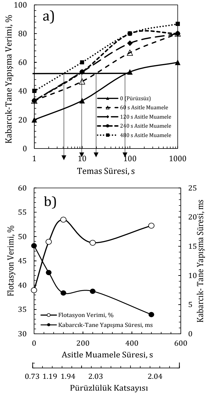
Şekil 3. a) Kabarcık-Tane Yapışma Verimine Bağlı Olarak Elde Edilen Temas Süreleri (%50 verimin elde edildiği süre yapışma süresi olarak adlandırılmaktadır) b) Asitle Muamele Süresine Bağlı Olarak Elde Edilen Pürüzlülük Katsayılarına Bağ Yuvarlak Pürüzlü Tanelerle Yapılan Kabarcık-Tane Yapışma Süresi Ölçümleri (Asitle Muamele Süreleri: 60, 120, 240, 480 sn)
