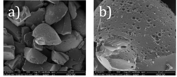
Şekil 7a. 240 s Asitle Muamele Edildikten Sonra Öğütülen Tanelerin 500x Büyütme Oranında S.E.M Görüntüsü b) 240 s Asitle Muamele Edildikten Sonra Öğütülen Tanelerin 2000x Büyütme Oranında S.E.M Görüntüsü
