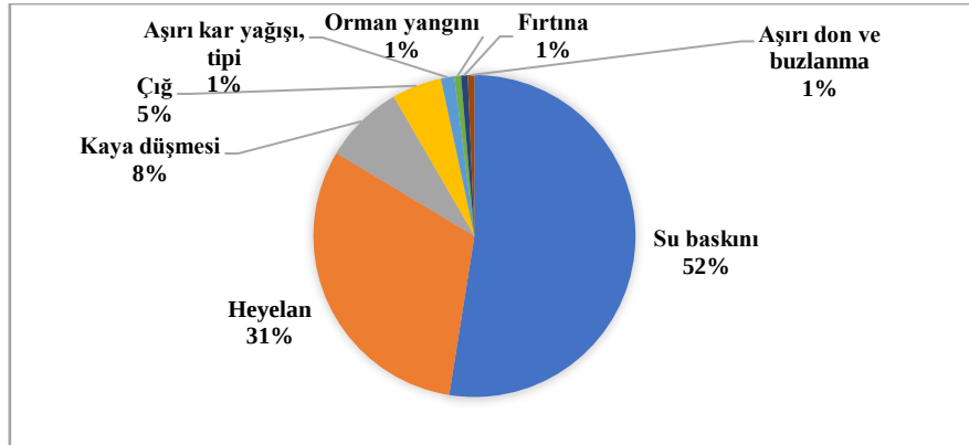
Şekil 3. Ağrı İli Sınırları İçerisinde 1975-2022 Dönemi Hava, İklim ve Su İle İlgili Afet Ve Olay Kaydı Sayısı (Kaynak: AYDES Bilişim Sistemi)
