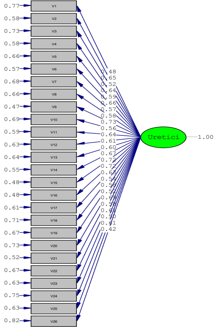
Şekil 4. Değişkenlerin Hata Varyansları
