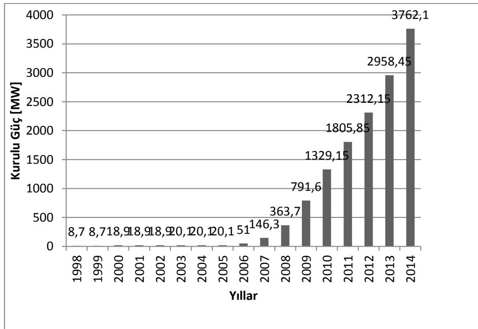
Şekil 3. Yıllara göre toplam rüzgar kurulu gücü
