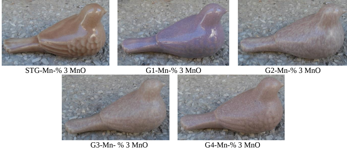
Şekil 5. Kalsit katkılı standart sırda mangan oksitin renk ve yüzey etkileri (1160 °C)
