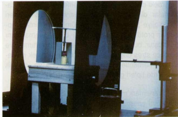
Şekil 4. Transmisyon polariskop cihazı
