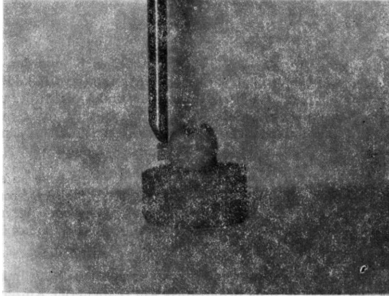
Resim 1: Kompozit-mine birleşim bölgesine çelik uç ile yük uygulanması.
