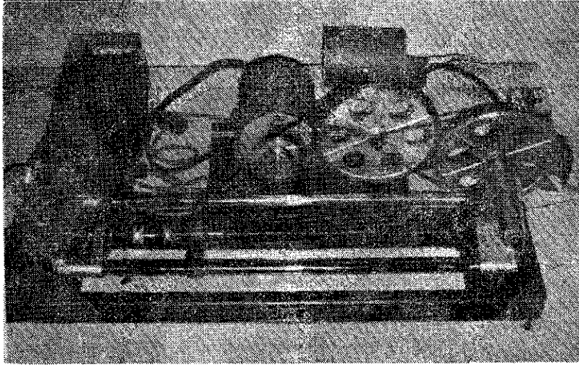
Resim 3. Hounsfield Tensometresi.
