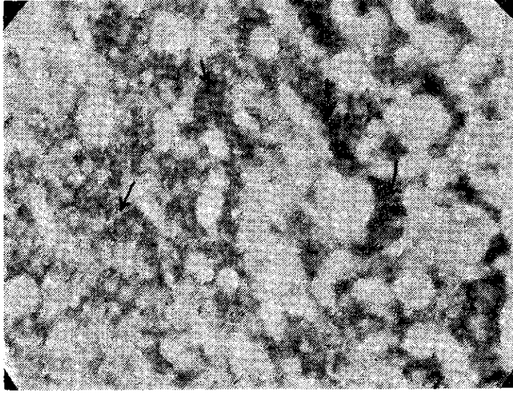
ŞEKİL 3. Dekzametazon verilmesinden sonra zona fasikolata hücreleri. Lipozomlardan zengin koyu hücreler okla işaretli. Sudan siyahı. X7.200
