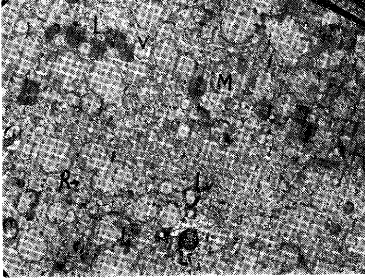
ŞEKİL 2. Kontrol kobay zona fasikülata hücresi. M : mitokondriyon, L : küçük homojen lipidler, Lv : ortası açık periferi elektroyoğun yapıdaki lipid, Li : lizozom, V : vakuol, R : ribozom.
