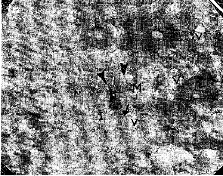
ŞEKİL 1. Kontrol kobay zona fasikülata hücresi. Laminar tipte kristallar gruplaşmalar göstermektedir. M : mitokondriyon, V : vakuol, R : ribzom, İ : interselüler aralık, L : lipid, Li : lizozom, Granül içeren mitokondriyon(ok), mitokondriyon-endoplazma retikulumu ilişkisi (okbaşı).
