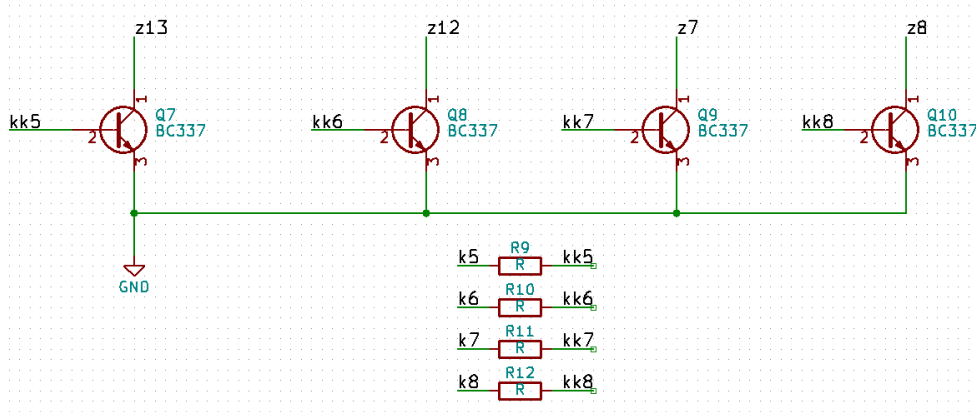
Şekil 5. Farklı pin dizilimine sahip entegrelerin GND bağlantıları
