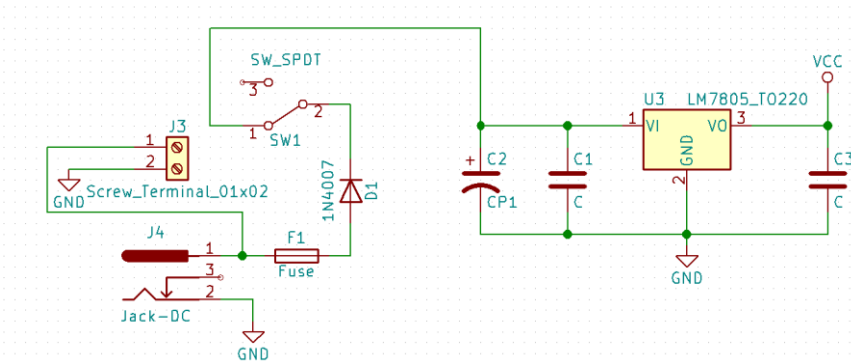
Şekil 2. Entegre test devresinin güç katı
