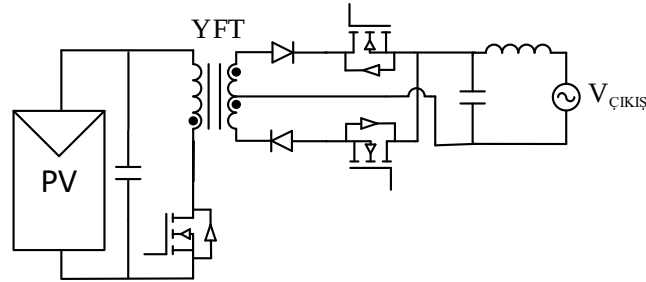
Şekil 8. Yüksek güç ayrıştırmalı flyback tipi evirici[65]
