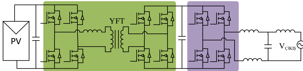
Şekil 9. Tam köprü DA/AA dönüştürücü[75]
