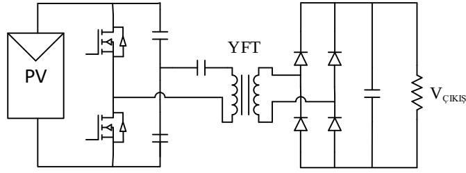
Şekil 14. Rezonans yarı köprü dönüştürücü [Hata! Başvuru kaynağı bulunamadı.]
