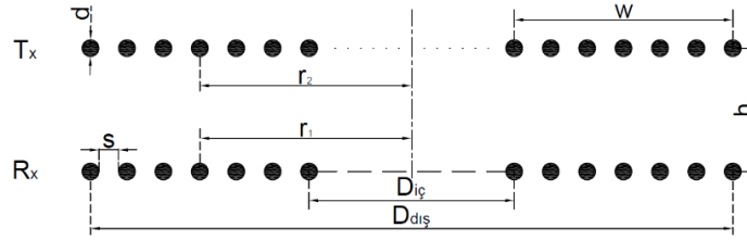
Şekil 2. Spiral dairesel bobin geometrisi
