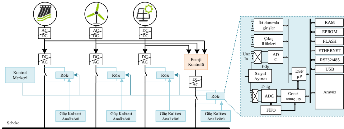
Şekil 4: Koruma fonksiyonlarını güç kalitesi analizi ile güç şebekesi bağlantı noktaları ve koruma rölesi analizörü
