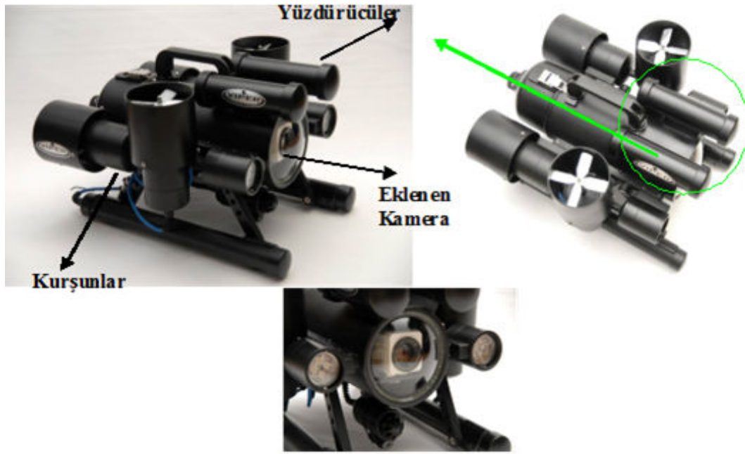
Şekil 5. Gövde tasarımıdaki değişiklikler (ön yüzdürücülerin eklenmesi, kurşun plakalarla denge ayarının yapılması)
