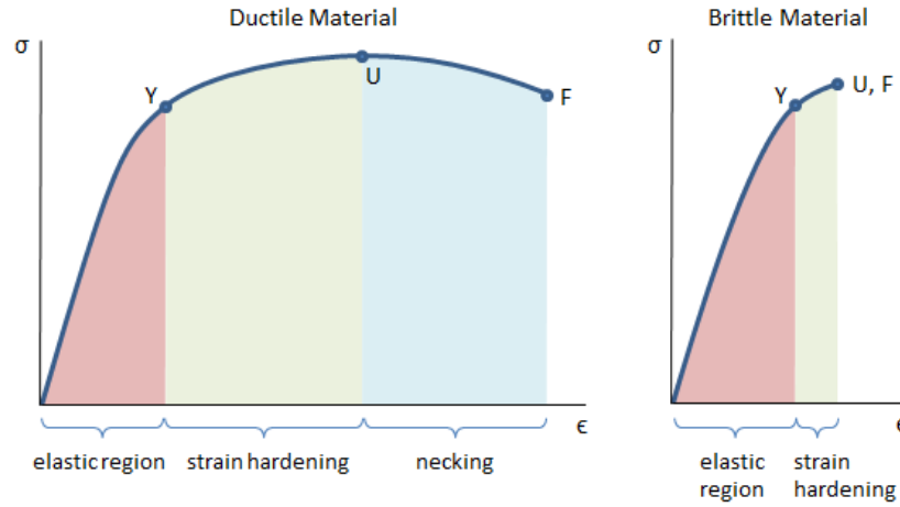
Figure 3. Comparison between ductile and brittle Stress & Strain diagram (Sünek ve kırılma malzemeler için gerilme-gerinim diyagramının karşılaştırılması) [24]
