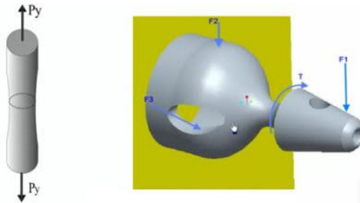
Figure 4. A simple tension test and a real-life loading condition (Basit bir gerilme testi ve gerçek hayat yükleme koşulu) [25]
