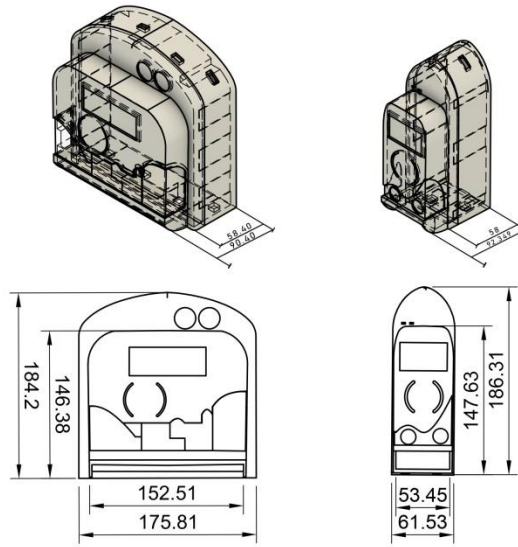
Figure 1. General dimensions of three-phase and monophase electricity meter products, wall thickness 3 mm (Trifaz ve monofaz elektrik sayacı ürünlerine ait genel ölçüler, et kalınlığı 3 mm)
