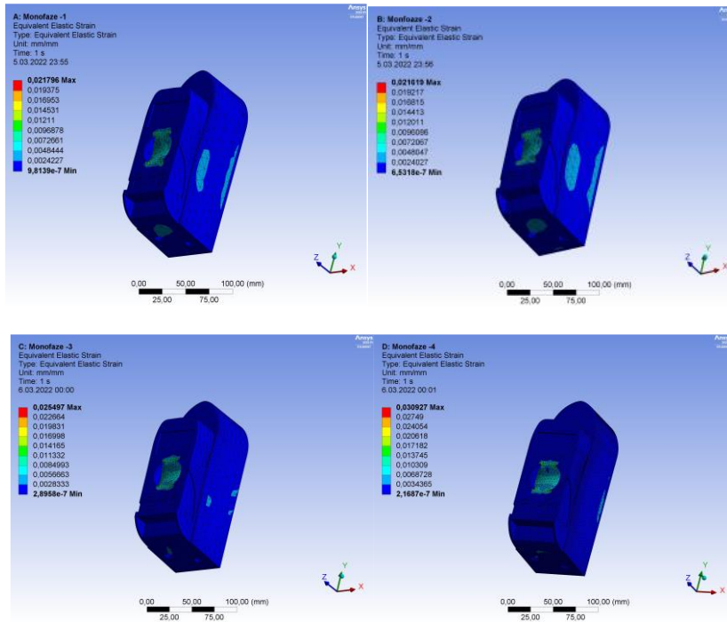
Figure 11. Total strain analyses for monophase (Monofaz için toplam gerinim analizi)
