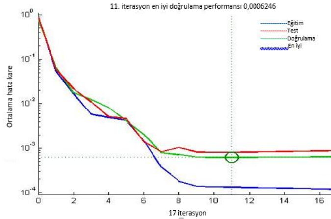
Şekil :5 Ağ Eğitim Hata Grafiği
