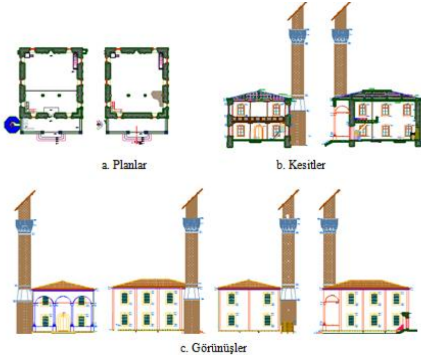
Şekil 3. Dürbinar Camisi kat planı, kesit ve cephe görünüşleri [19]. (Dürbinar Mosque’s side view and floor plans)
