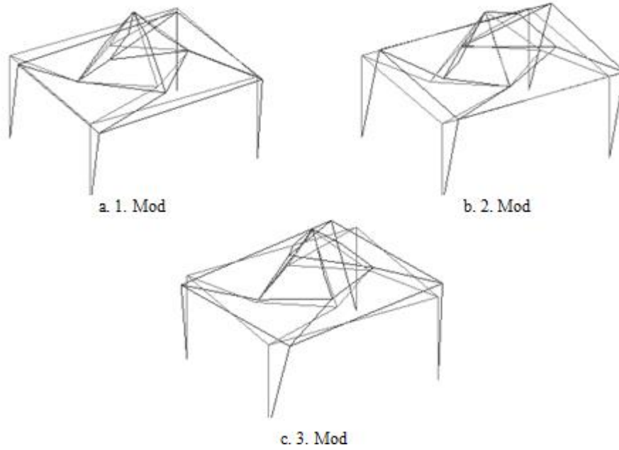
Şekil 9. Dürbinar Camisinin restorasyon öncesi durumuna ait ilk üç deneysel mod şekli (First three mode shapes of Dürbinar Mosque before the restoration)
