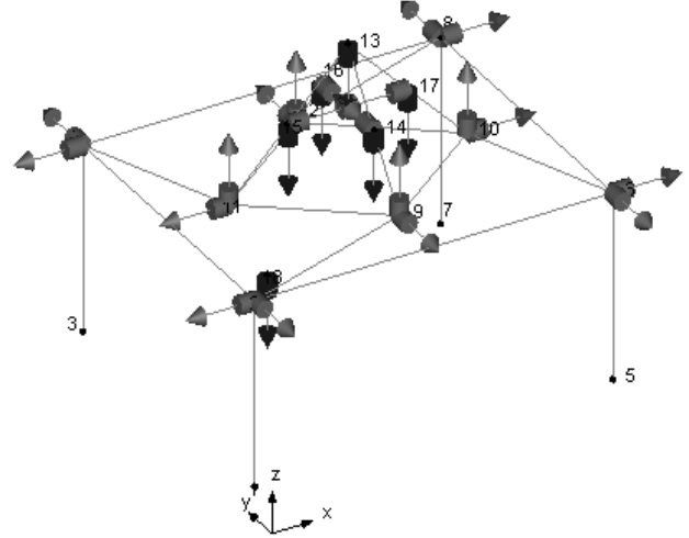
Şekil 7. Dürbinar Camisindeki restorasyon öncesi ivmeölçer yerleşim düzeni
