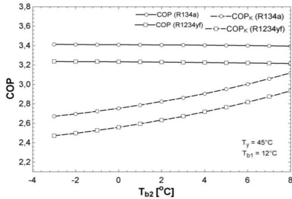
Şekil 11. İkinci buharlaştırıcı sıcaklığının soğutma etkinliği üzerine etkisi (The effect of second evaporator temperature on coefficient of performance)
