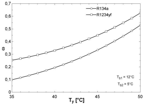
Şekil 7. Yoğuşturucu sıcaklığının kütleli debi oranı üzerine etkisi (The effect of condenser temperature on entrainment ratio)
