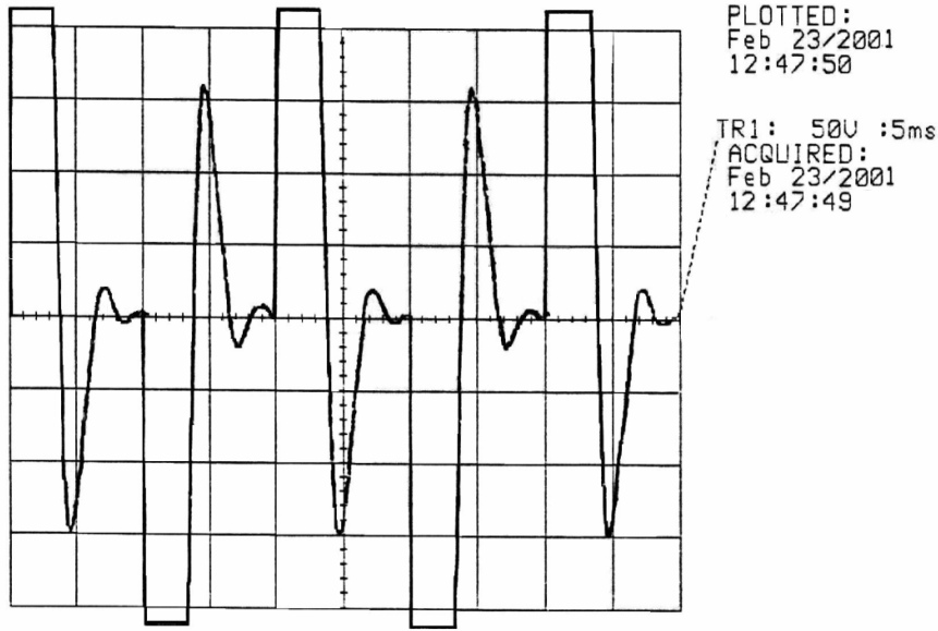
Şekil 3. Kesintisiz güç kaynağının çıkış sinyali
