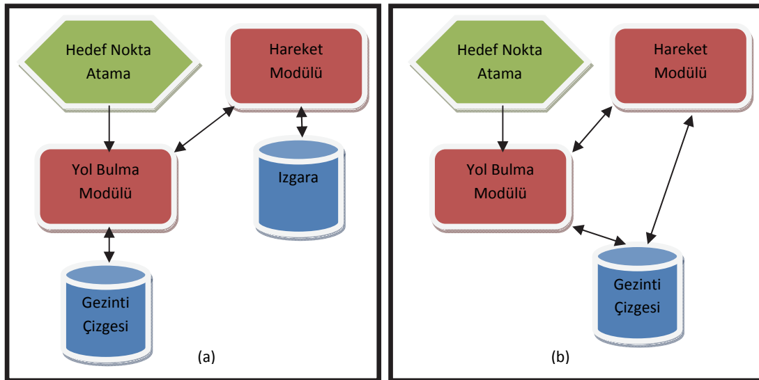
Şekil 1. (a) İzgara tabanlı çalışan sistemin genel yapısı. (b) Önerilen çizge tabanlı sistemin genel yapısı. (a) General structure of the grid based system. (b) General structure of the proposed graph based system.)
