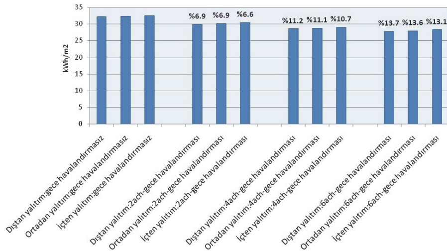
Şekil 7. Gece havalandırması performansına yalıtım yeri ve hava hızının etkisi-2050(The effect of insulation location and air flow rate on performance of night ventilation-2050)
