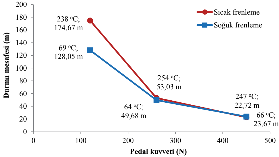
Şekil 8. Fren disk sıcaklığının durma mesafesine etkisi, 60 km/h ve yüksüz (The effect of brake disc temperature on stopping distance, 60km/h and unladen)
