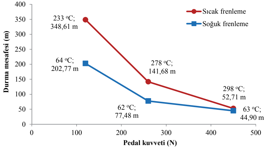
Şekil 4. Fren disk sıcaklığının durma mesafesine etkisi, 80 km/h ve yüklü (The effect of brake disc temperature on stopping distance, 80 km/h and laden)
