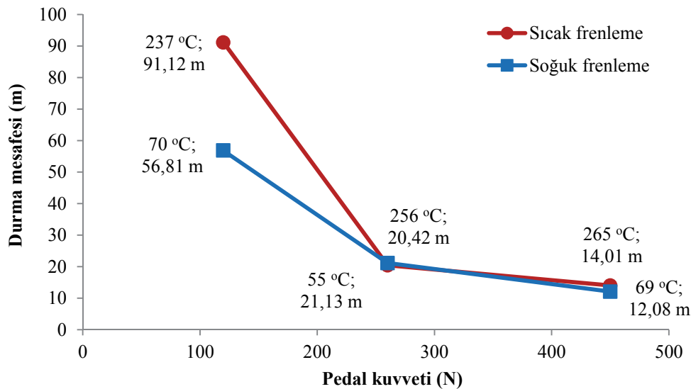
Şekil 9. Fren disk sıcaklığının durma mesafesine etkisi, 40 km/h ve yüksüz (The effect of brake disc temperature on stopping distance, 40 km/h and unladen)
