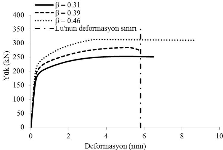
Şekil 10. Çok düzlemli K-birleşimlerinin yük- deformasyon grafiği
