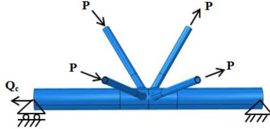
Şekil 7. Sayısal modellerin mesnet sınır koşulları ve yükleme durumu
