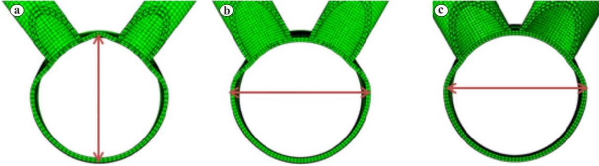
Şekil 9. Çok düzlemli K-birleşimlerin deformasyonları. (a) \beta = 0.31 . (b) \beta = 0.39 . (c) \beta = 0.46
