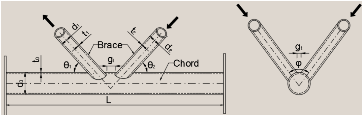
Şekil 2. Çok düzlemlî K-birleşiminin geometrik parametreleri
