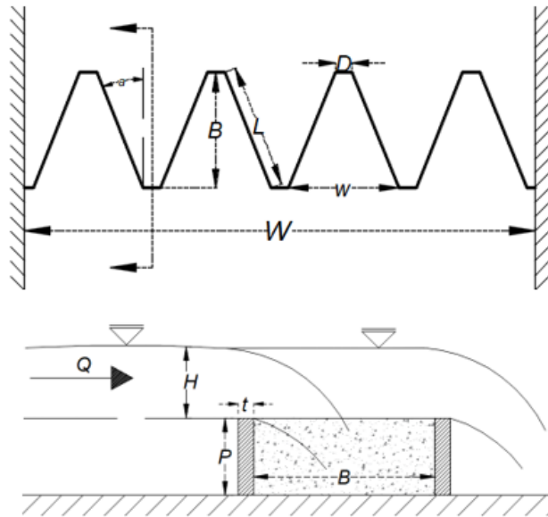
Şekil 5. Labirent savaklarda akımı etkileyen parametreler
