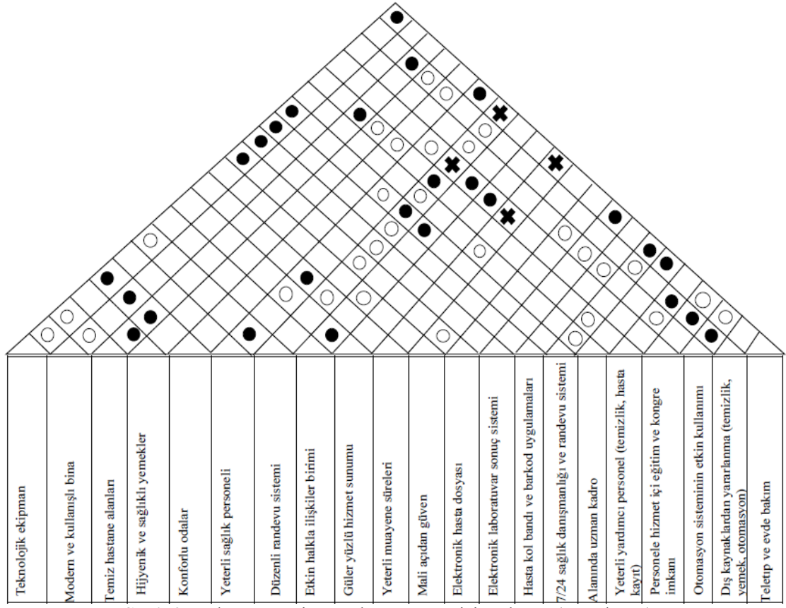
Şekil 9. Çalışmaya Ait Korelasyon Matrisi Bölümü (E Bölümü)
