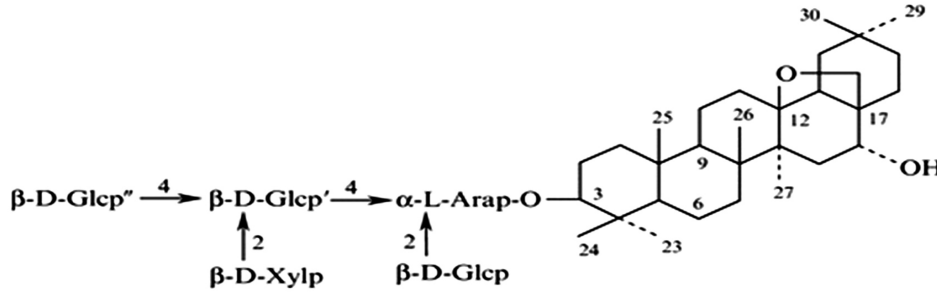
Şekil 3 Anagalloside
