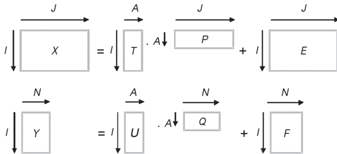
Şekil 2 PLS2 kalibrasyonu
