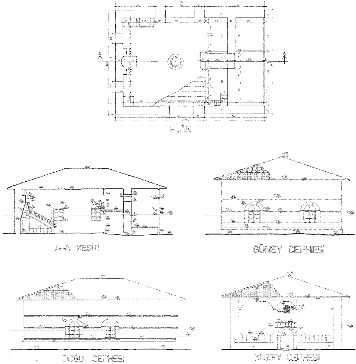
Plan 1: Sakarca Köyü Camisi Planı, Kesiti ve Cephe Çizimleri (Vakıflar Genel Müdürlüğü Arşivi'nden, 2015)
