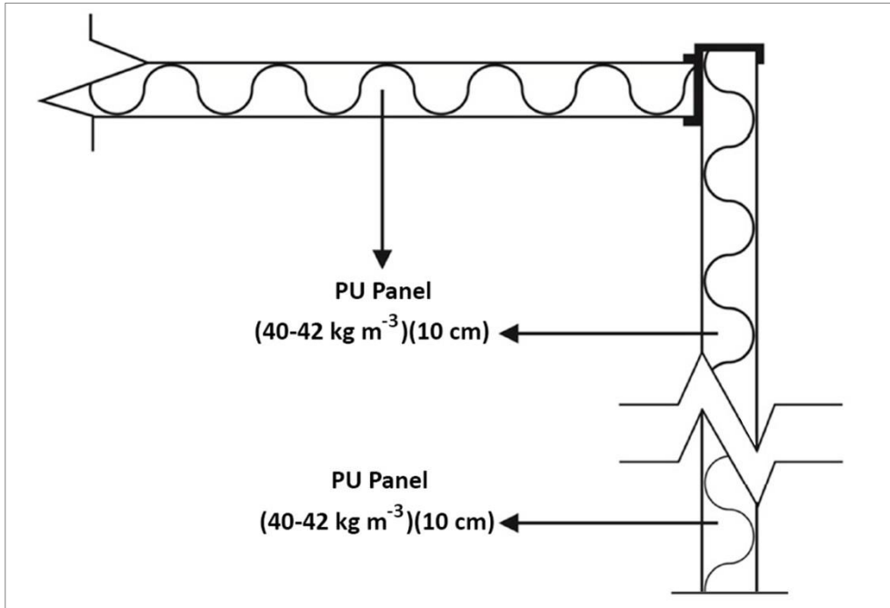
Şekil 3. Poliüretan panel kullanılan depounun duvar ve tavan detayı (Yılmaz ve ark., 2017)
