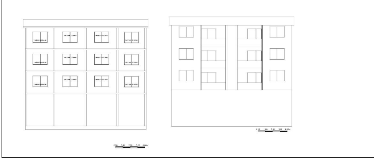
Şekil 32. Ökkeş Abasıkeleş Apartmanı; Sol A-A Kesit Planı, Sağ Ön Görünüş Planı (Osmaniye Belediyesi 2022).
