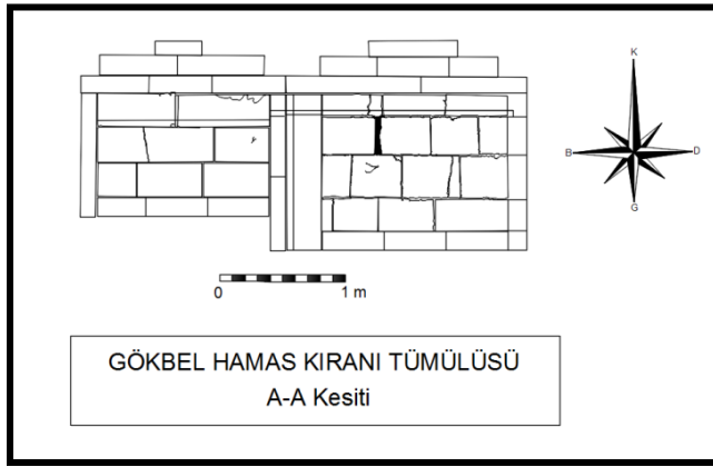
Çizim 1: Hamas Kırani Tümülüsü altı mezar yapısının A-A kesiti(G. Laçın, Ş. Yıldırım).
