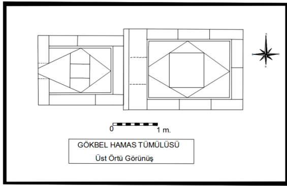
Çizim 2: Hamas Kıranı Tümlüsü ön oda ve asıl mezar odası üst örtüsü görünüş(Ş. Yıldırım, G. Laçın).
