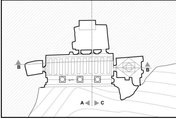
Çizim 6: Karakoyunlu kaya mezarının planı ve aykırı taşı rma teknikli mezar odasının tavanı(Çizen: Mümtaz Beyazođlu).
