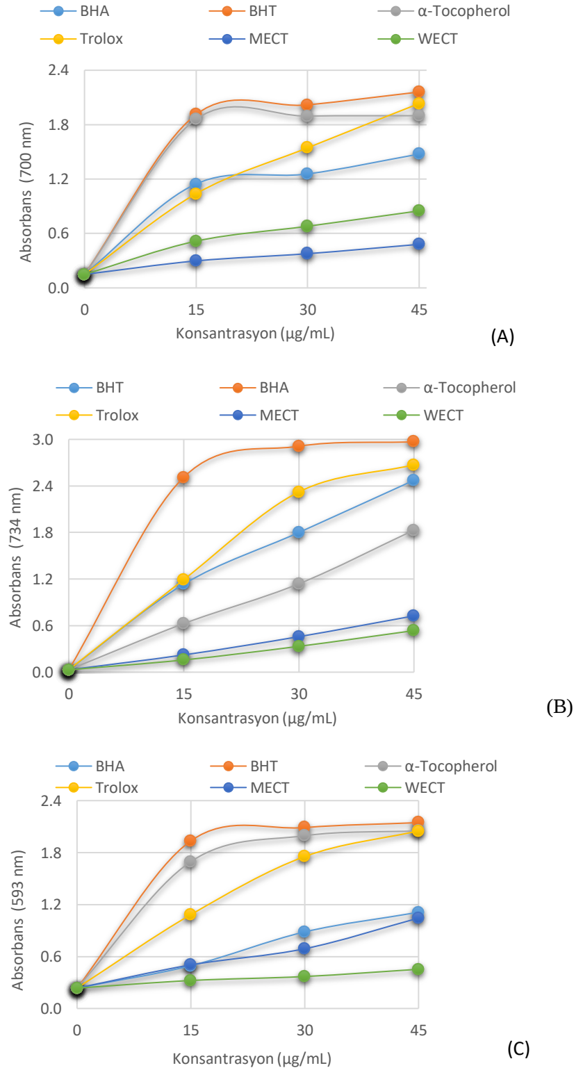
Şekil 2. Cephalaria ekstrelerinin A. Fe 3+ indirgeme, B. Cu 2+ indirgeme and C. Fe 3+ -TPTZ indirgeme kabiliyetleri
