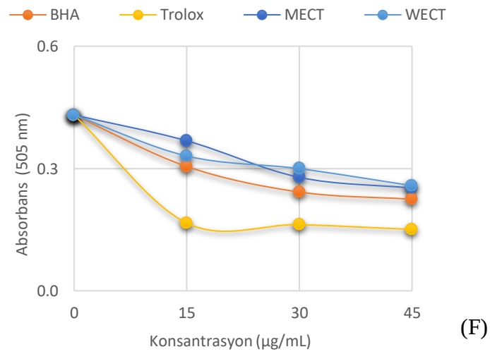
Şekil 3. Cephalaria ekstrelerinin ve standartların radikal süpürücü etkileri. D. DPPH• süpürücü yetenek, E. ABTS•+ süpürücü yetenek, F. DMPD•+ süpürücü yetenek
