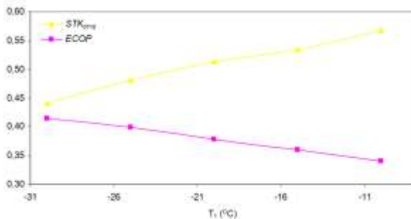
Şekil 2. Açık ara soğutuculu buhar sıkıştırma-absorbsiyonlu çift kademeli soğutma çevriminin STK_{cevg} ve ECOP değerlerinin buharlaştırıcı sıcaklığı ( T_1 ) ile değişimi.
