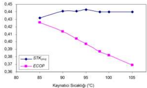
Şekil 4. STK_{cevg} ’nin kaynatıcı sıcaklığı ile değişimi.
