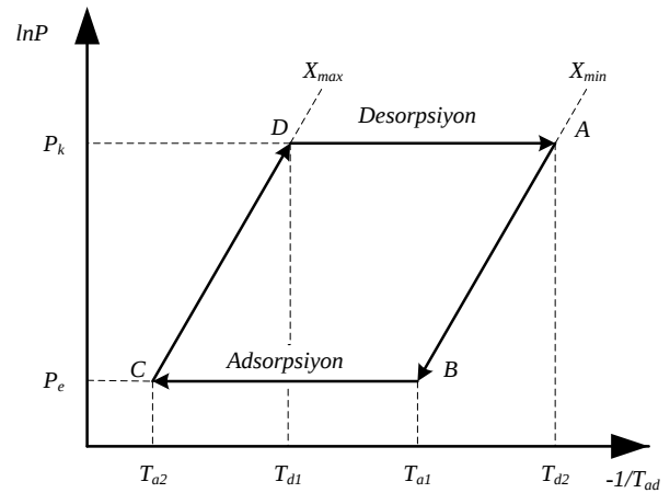
Şekil 2. Clapeyron diyagramı.
