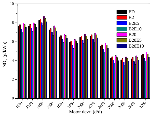
Şekil 11. Biyodizel-dizel yakıt karışımlarına etanol ilavesinin NO x emisyonu üzerine etkisi
