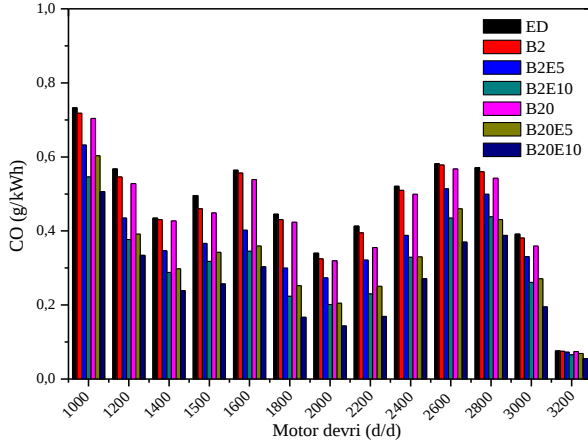
Şekil 8. Biyodizel-dizel yakıt karışımlarına etanol ilavesinin CO emisyonu üzerine etkisi
