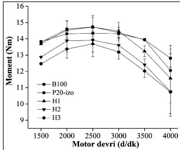
Şekil 5. P20-izo yakıtına farklı miktarlarda ilave edilen hekzan'ın motor momentine etkisi
