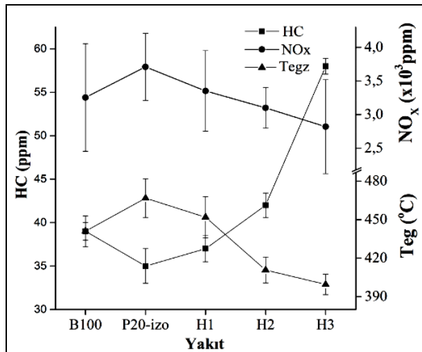
Şekil 8. P20 izo yakıtına farklı miktarlarda ilave edilen hekzanın maksimum motor gücü devrinde HC, NO x ve ve egzoz gaz sıcaklığına etkisi
