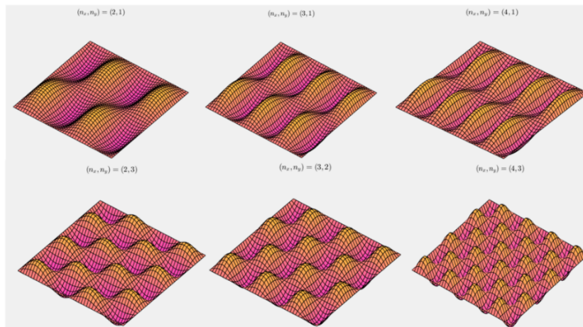
Şekil 4. Üretilen altı-mod değeri için dikdörtgensel düzlem yüzeyin titreşim grafikleri görülmektedir
