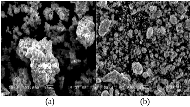
Şekil 1. a) Aktive edilmemiş; b) Mekanik olarak aktive edilmiş konsantrenin SEM görüntüleri.
