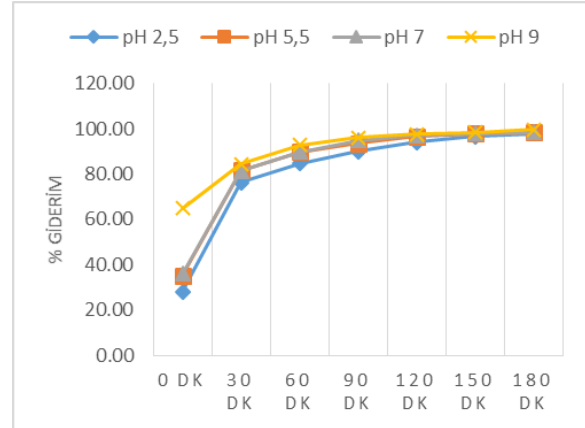
Şekil 8. ZnO'nun renk giderim verimine pH'nın etkisi.
