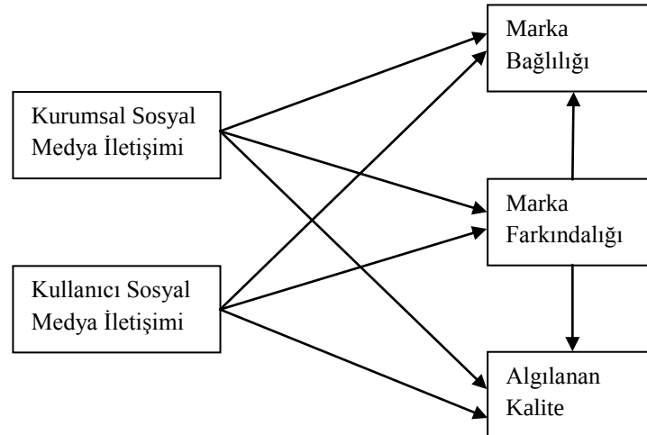
Şekil 1. Araştırmanın Modeli
