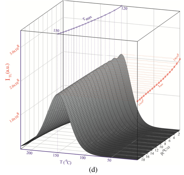
Şekil 3 n_o (a), E_e (b), s (c) ve \beta (d) parametrelerinin T_{\text{maks.}} ve I_{\text{maks.}} üzerindeki etkileri
