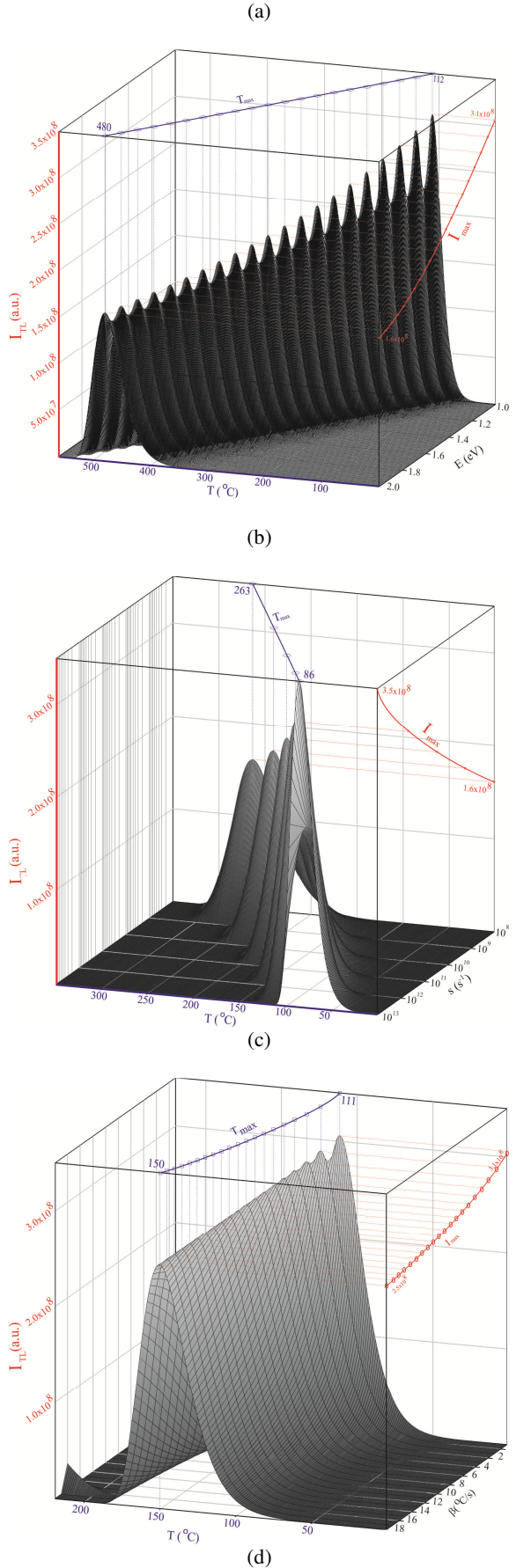
Şekil 4 n 0 (a), E e (b), s (c) ve β (d) parametrelerinin T max ve I max üzerindeki etkileri
