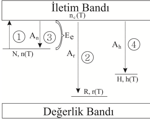
Şekil 1 Temel termoluminesans modeller için enerji-bant diyagramı
