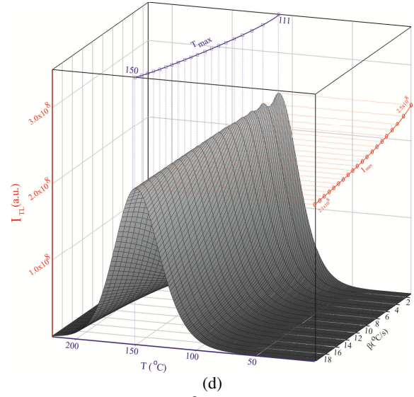
Şekil 4 n_o (a), E_c (b), s (c) ve \beta (d) parametrelerinin T_{maks.} ve I_{maks.} üzerindeki etkileri
