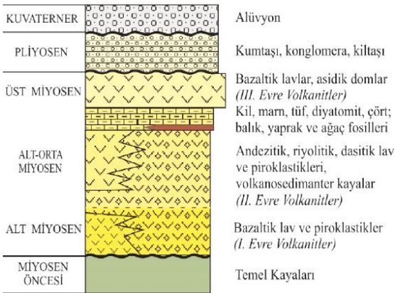
Şekil 4. Kızılcahamam-Çamlıdere bölgesindeki kayaçların stratigrafik dizilişi
