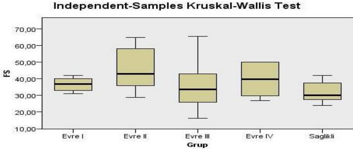
Şekil 4. FS parametresinin gruplara göre dağılımına ilişkin kutu grafiği
